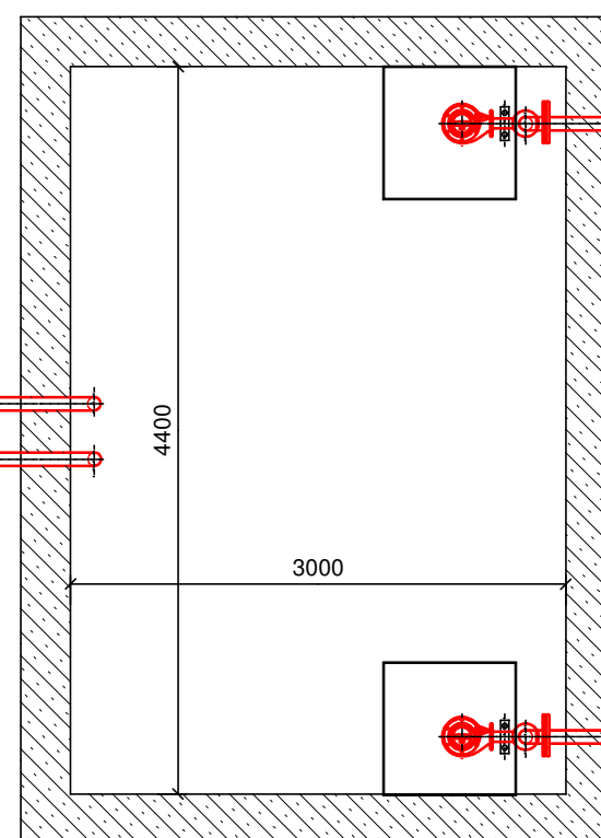
VYROVNÁVACIA NÁDRŽ
